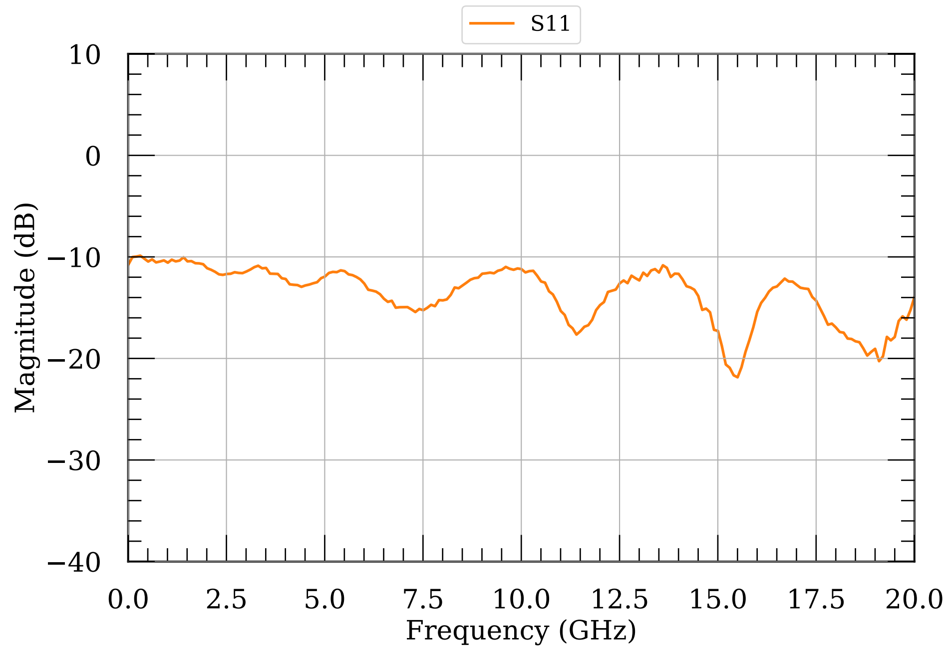
LNA S-params module003
